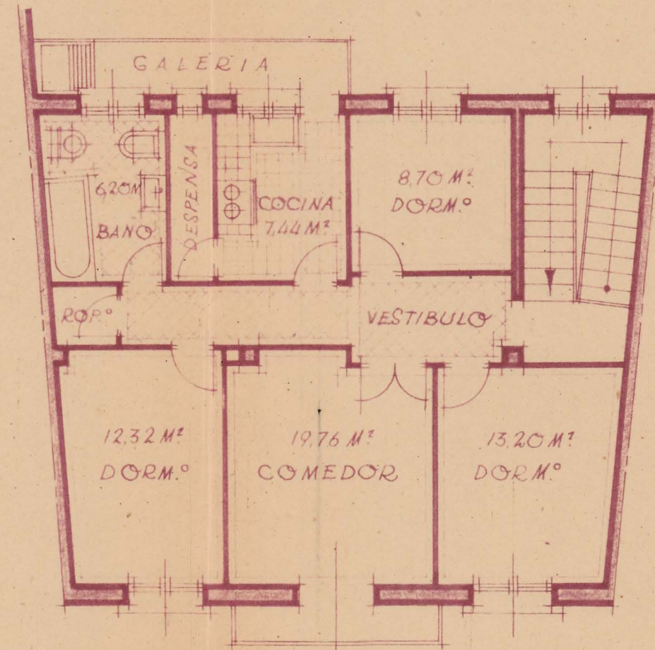
planta 2ª
