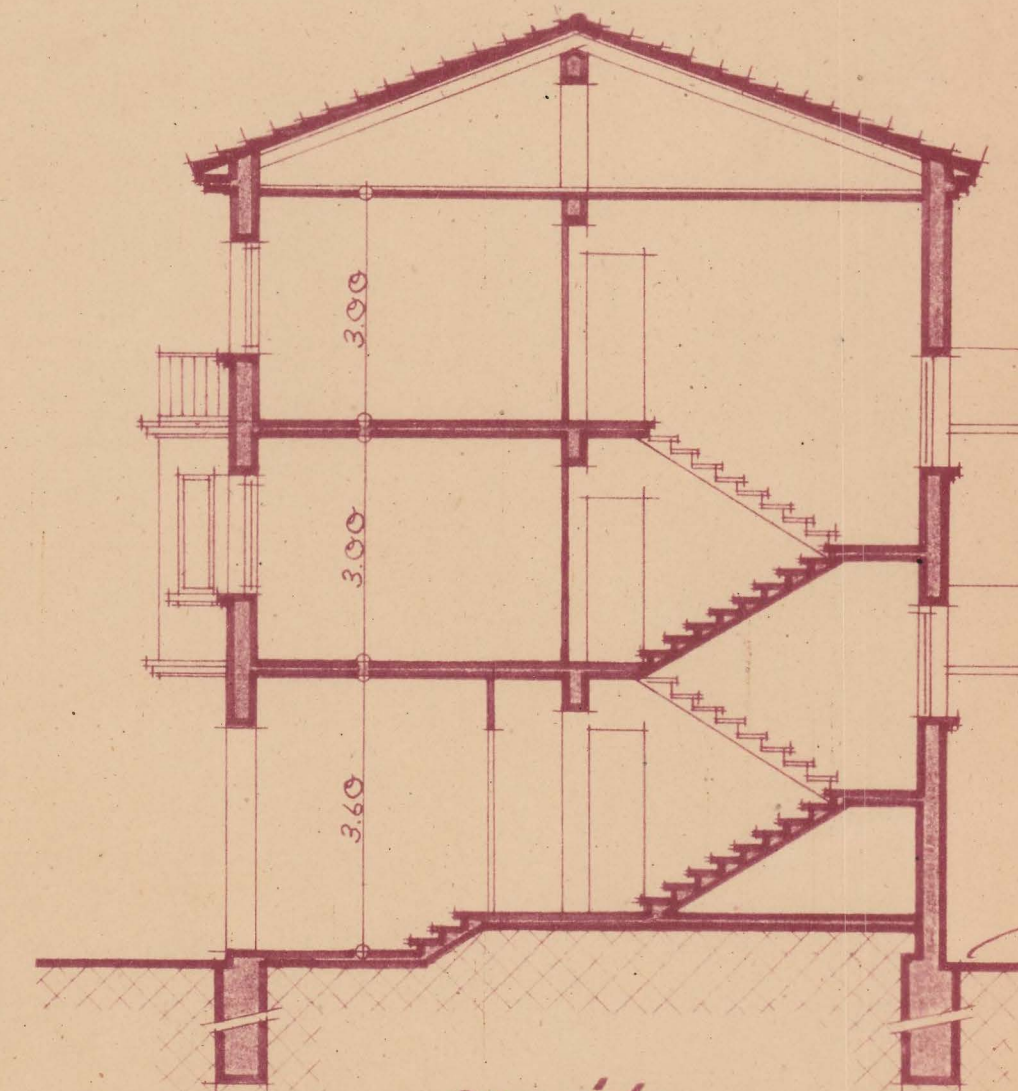
sección
