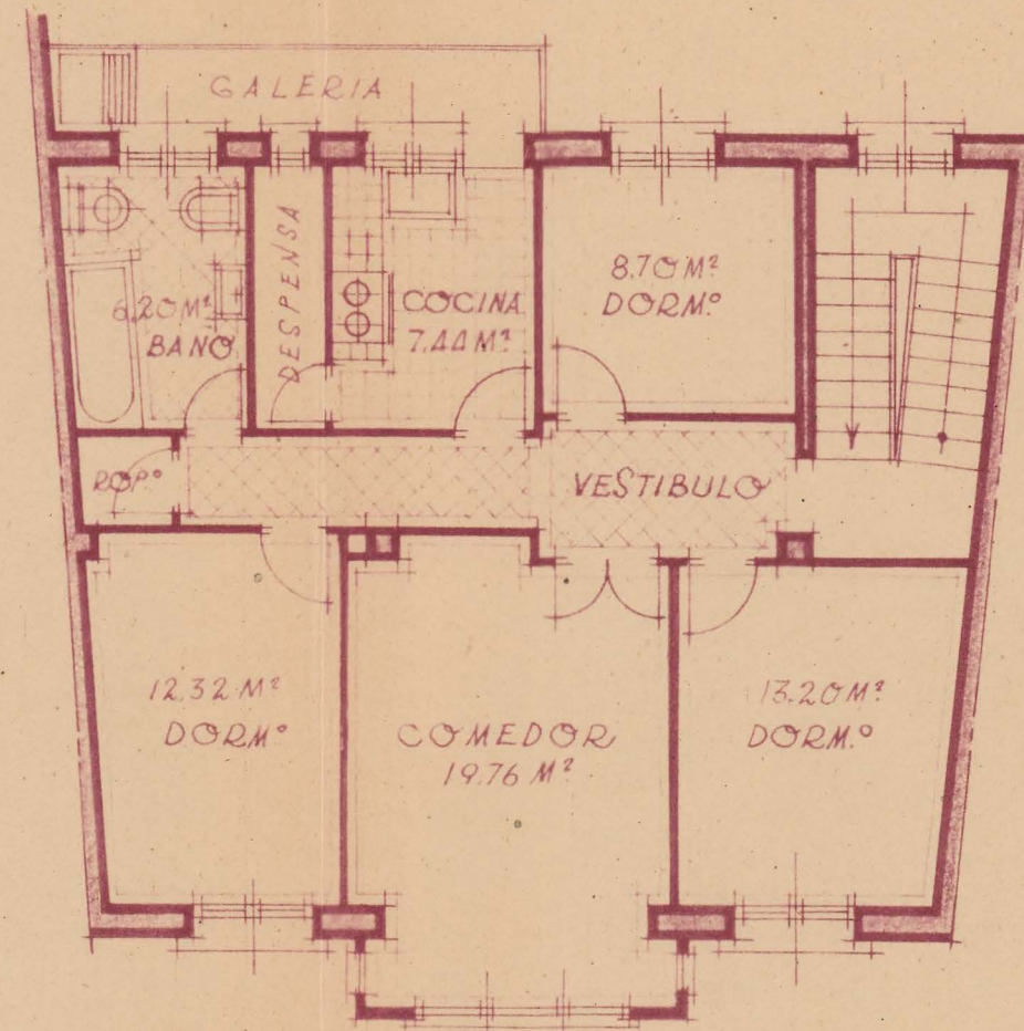
planta 1ª
