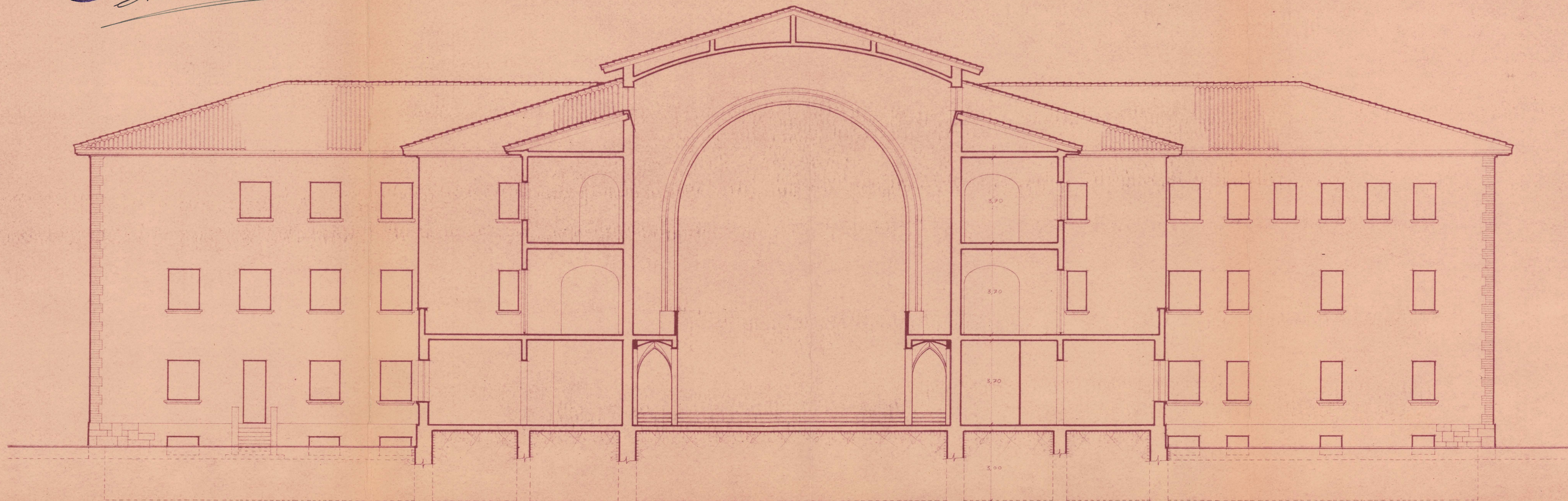
SECCION A-B.
