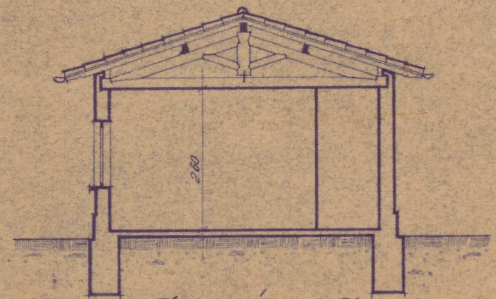
Sección A-B
