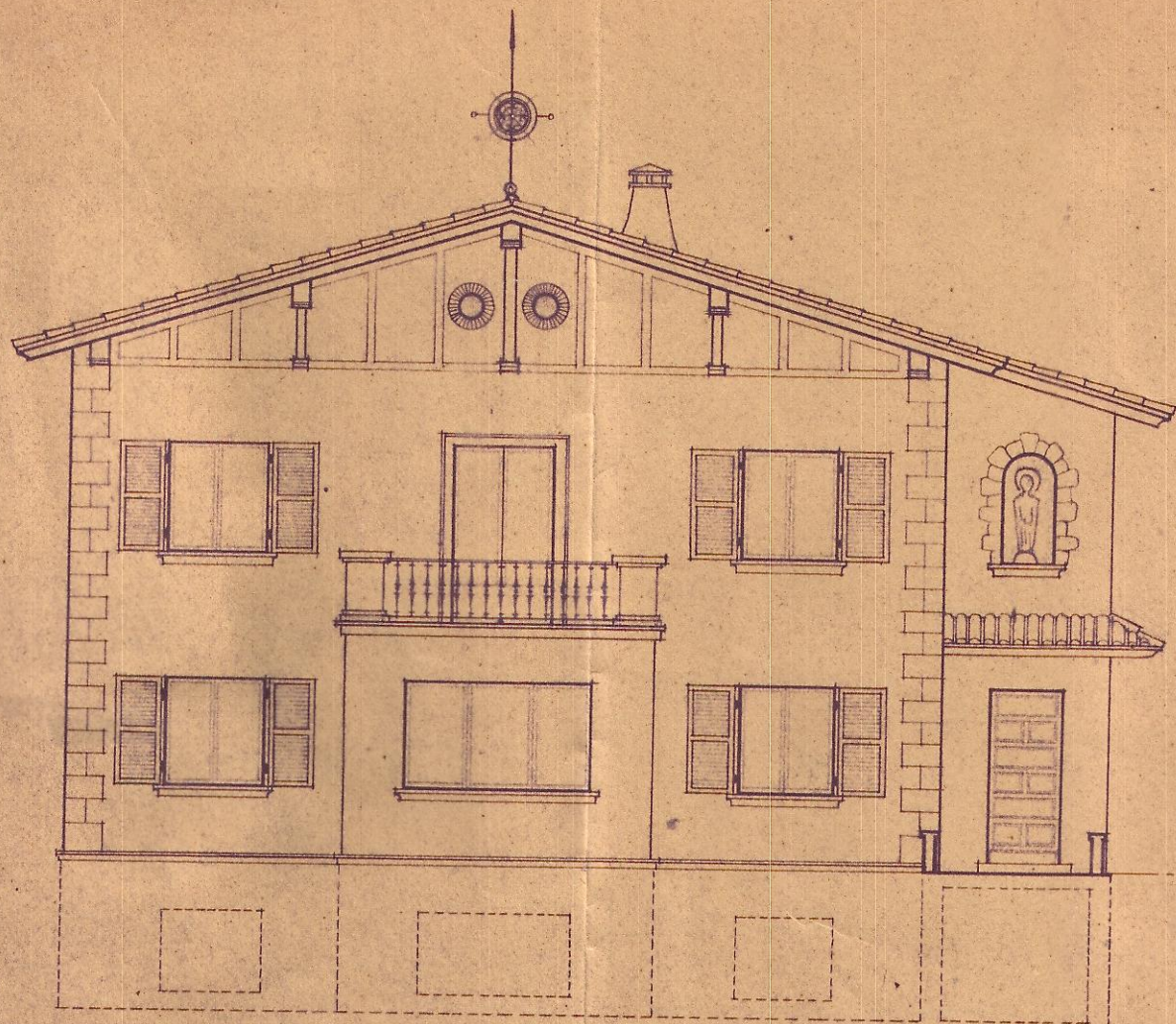
• Alzado principal •
