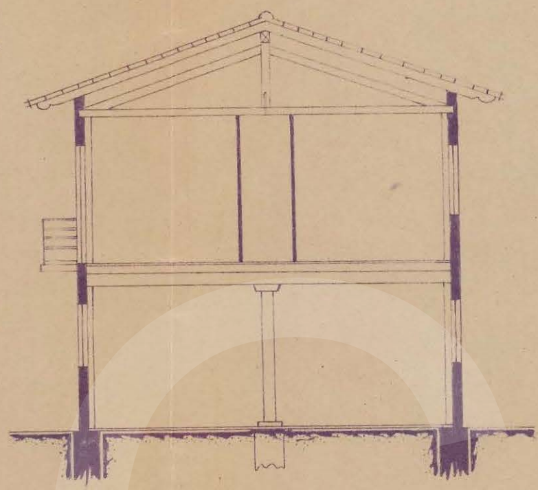
SECCION
