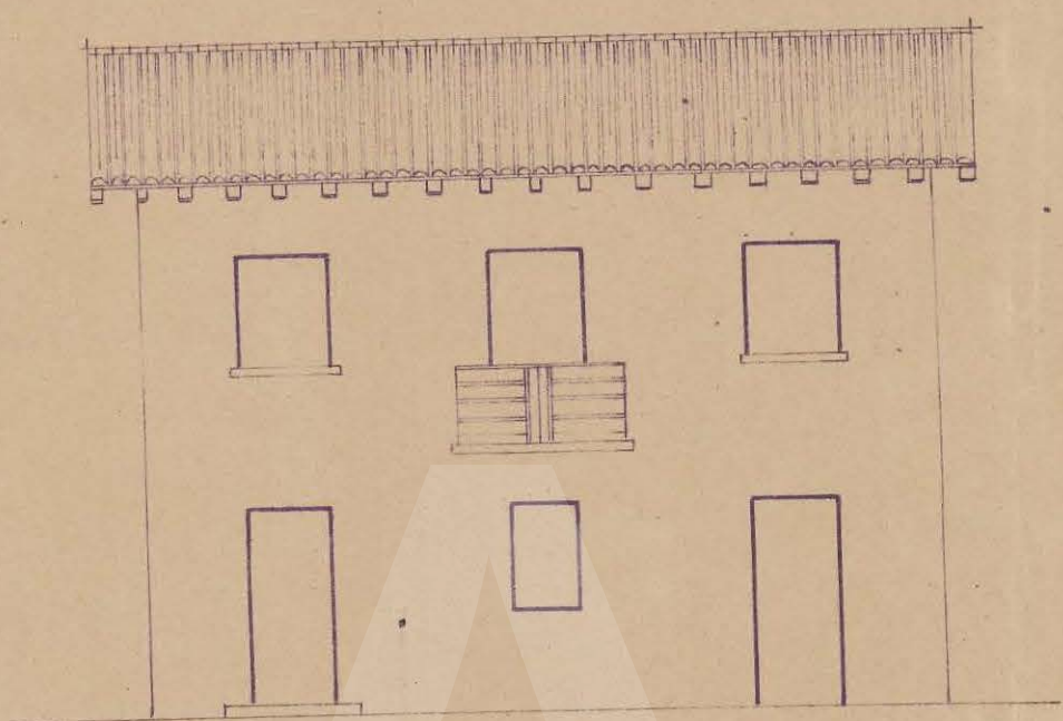
FACHADA
