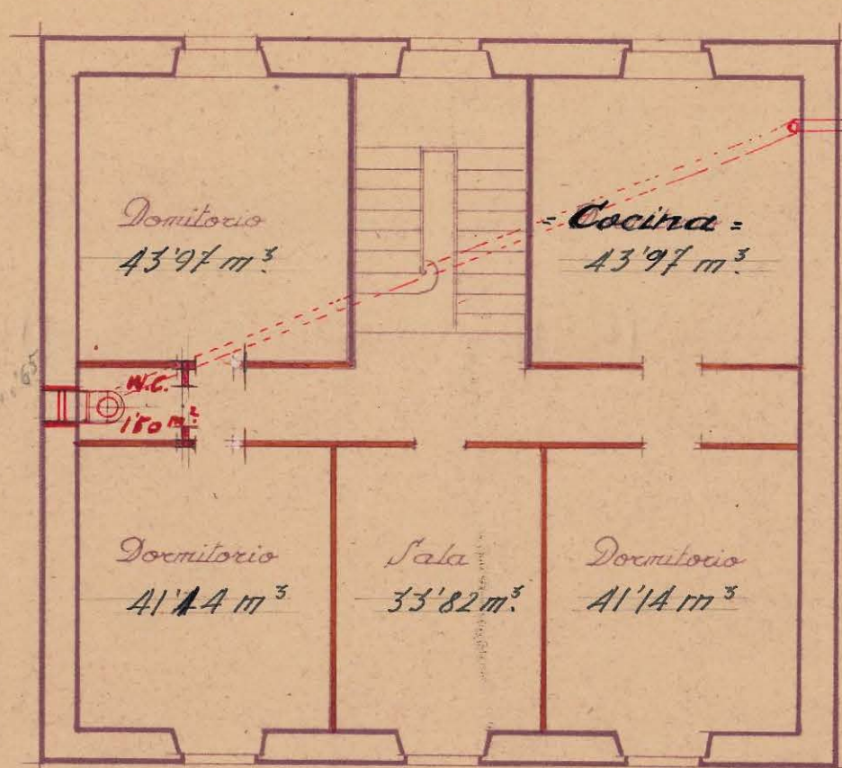
Planta principal
