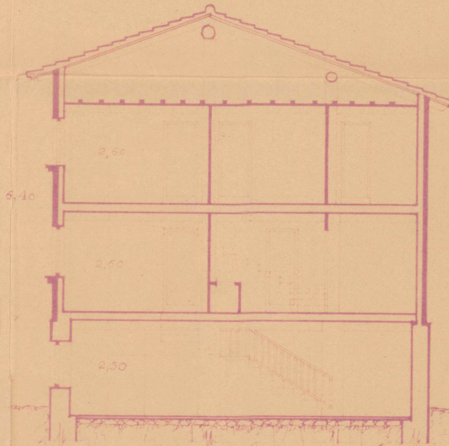
Sección A.B.
