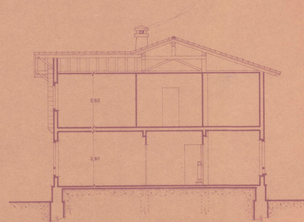
SECCION A-B
