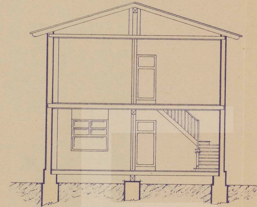
SECCION A.B.
